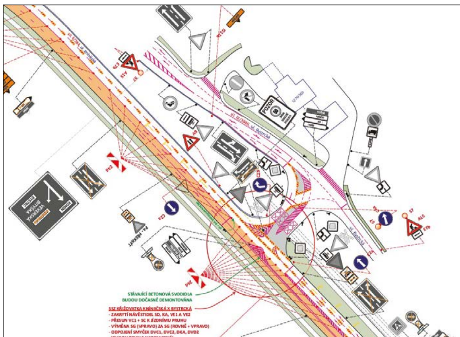
Detail křižovatky Kníničská x Bystrcká
